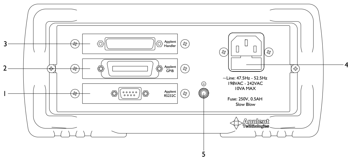
图 3-5 后面板(后面板示意图可能与实际位置不符)
