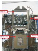
Vista del socket 1155-Pin
