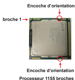
Processeur 1155 broches
