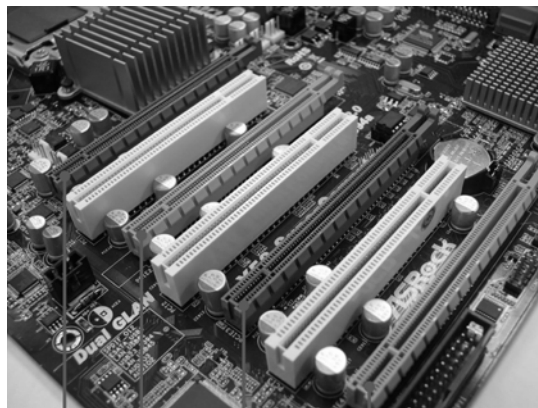
PCIe1 插槽 (x16 或 x8 模式)
