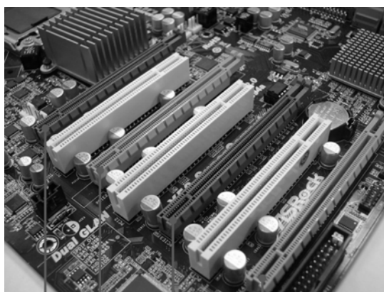
Alloggio PCIe1 (modalità x16 o x8)
