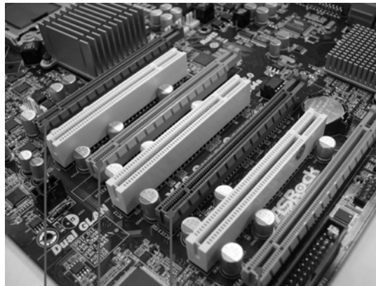
PCIE1 슬롯 (x16 또는 x8 모드)
