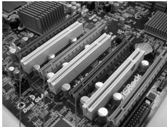
PCIE1 スロット (x16 または x8 モード)
