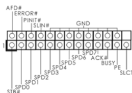
印表機接針 (25 針 LPT1) (見第 2 頁第 23 項)
