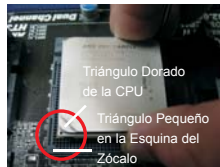
PASO 2 / PASO 3: Encaje el Triángulo Dorado de la CPU Con el Triángulo Pequeño de la Esquina del Zócalo
