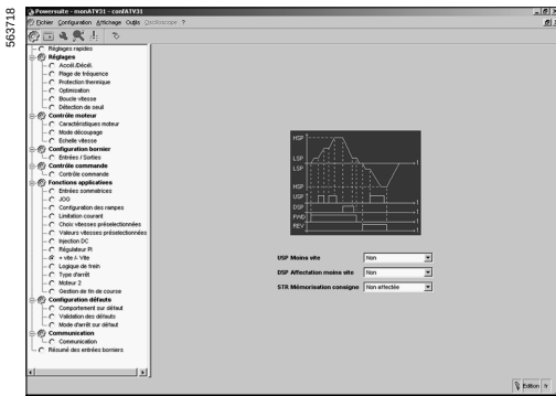
使用 PowerSuite for PC 调整 +/- 速度功能
