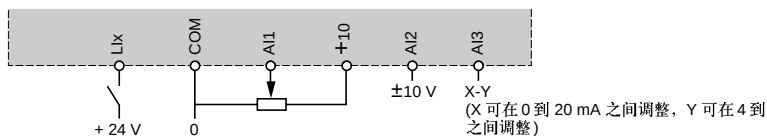
给定切换的连接图
