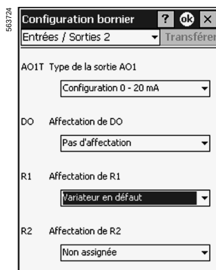
使用 PowerSuite for Pocket PC 对故障继电器的配置
