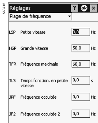
使用PowerSuite for Pocket PC 调整频率
