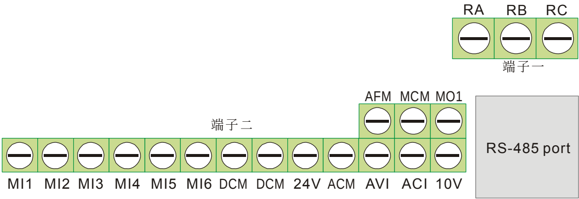
控制端子位置图
