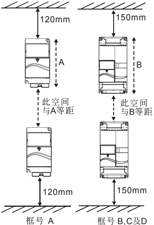
无分隔板设置图
