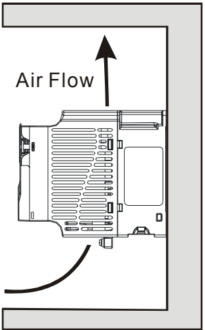
侧面通风设置图
