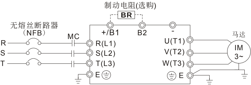
主回路端子图三
