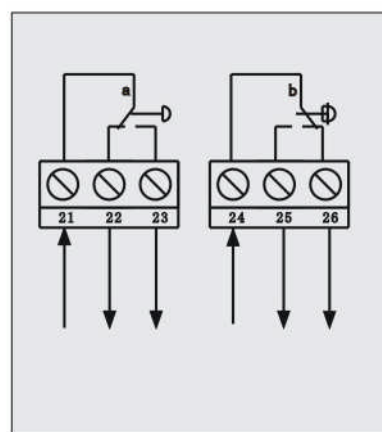
带辅助触点接线图
