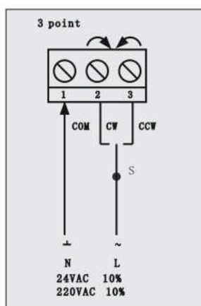
A9006 / A9009 接线图
