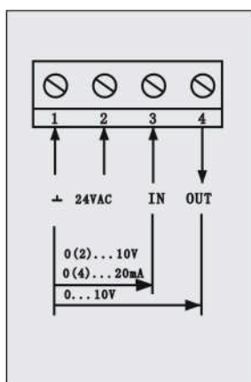
A9106 / A9109 接线图
