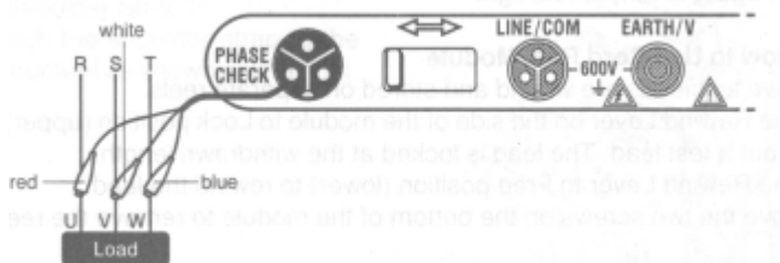
图 10 相位测量
