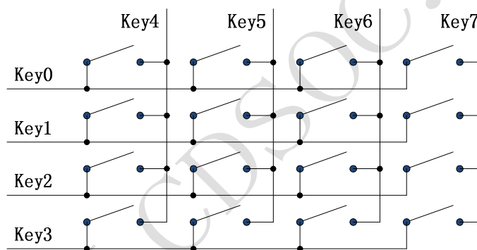
图 矩阵按键示意图
