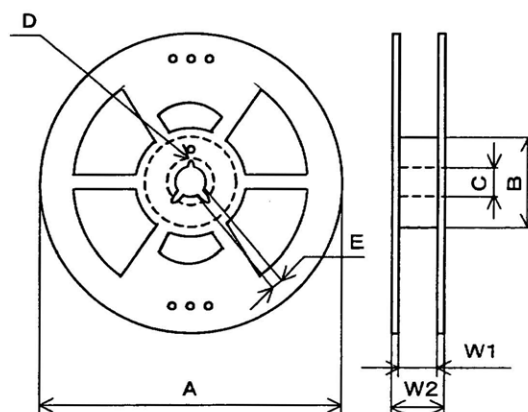
Fig. 4 Reel dimensions
