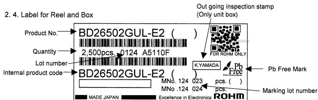
Fig. 5 Label example
