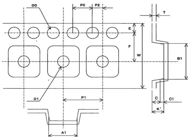
Fig. 3 Tape dimensions
