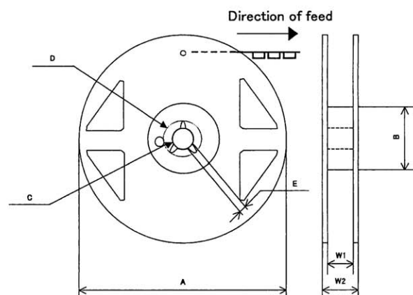
Fig. 4 Reel dimensions
