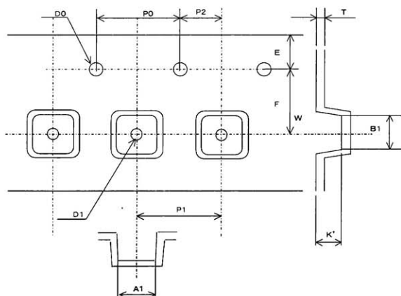
Fig. 3 Tape dimensions
