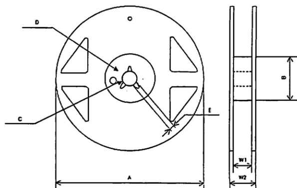
Fig. 4 Reel dimensions
