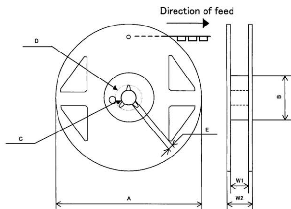
Fig. 4 Reel dimensions
