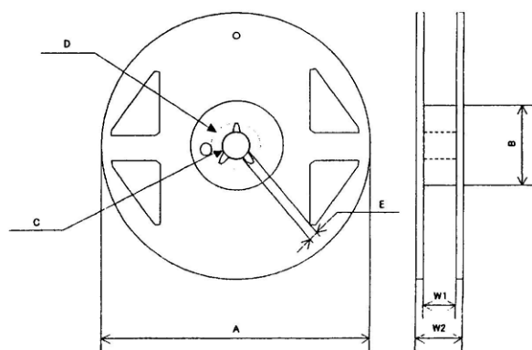
Fig. 4 Reel dimensions
