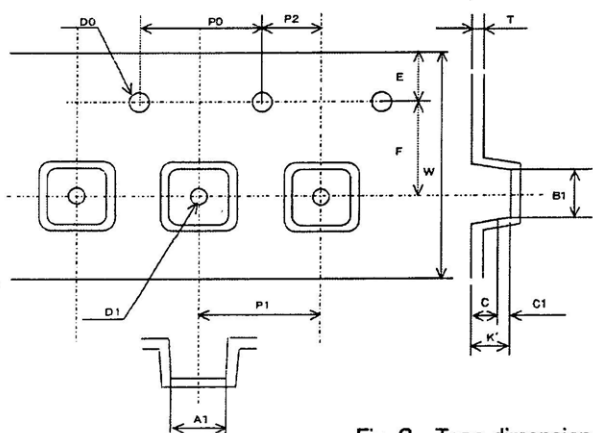
Fig. 3 Tape dimensions
