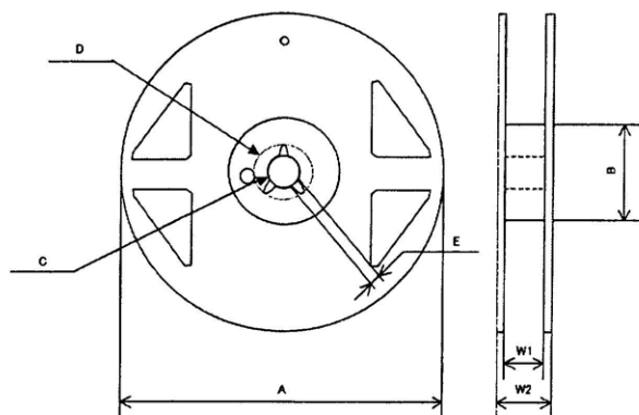
Fig. 4 Reel dimensions
