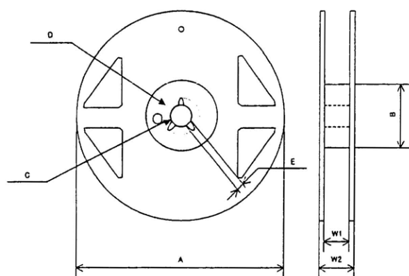
Fig. 4 Reel dimensions
