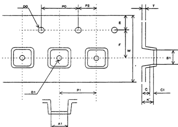
Fig. 3 Tape dimensions
