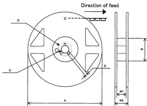
Fig. 4 Reel dimensions
