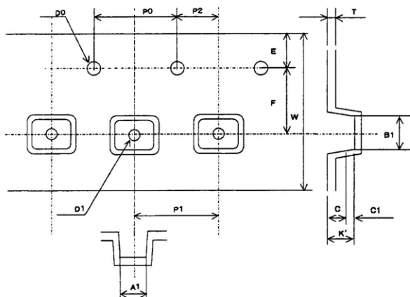
Fig. 3 Tape dimensions
