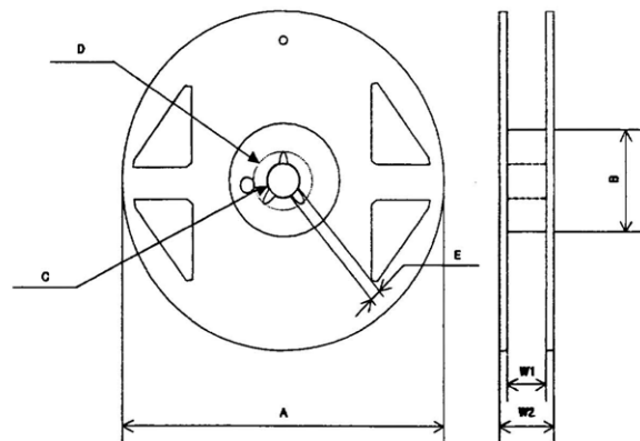
Fig. 4 Reel dimensions
