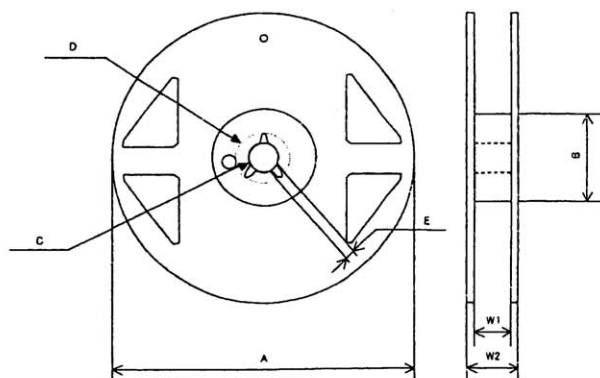
Fig. 4 Reel dimensions
