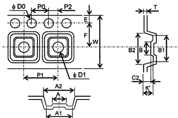
Fig. 3 Tape dimensions
