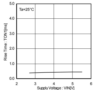
Fig.19 Output rise time
