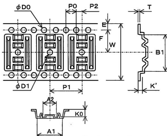
Fig. 3 Tape dimensions
