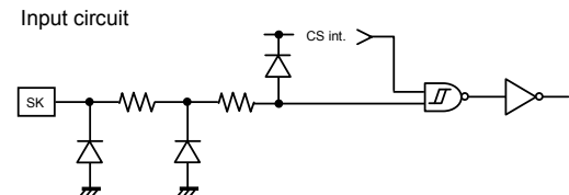
Fig.43 Input circuit (SK)
