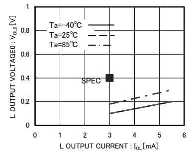
Fig.10 'L' Output Voltage0 V_{OL0-IOL} ( V_{CC0}=3.0V )
