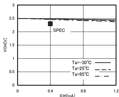
Fig.10 "H" output voltage VOH
