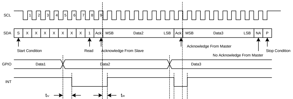
Fig. 17 Interrupt Valid/Reset
