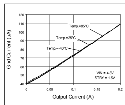
Fig. 16 IOUT - IIGN
