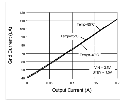
Fig. 71 IOU - IGND
