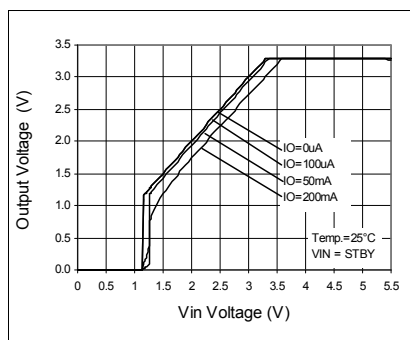
Fig. 11 Output Voltage
