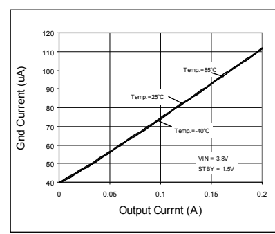
Fig. 45 IOOUT - IIGND
