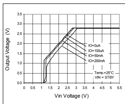
Fig. 40 Output Voltage
