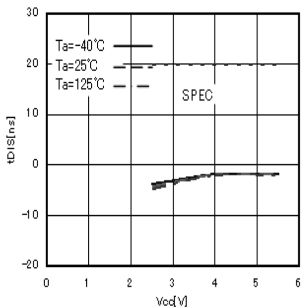
Fig.21 SI setup time t_{DIS}
