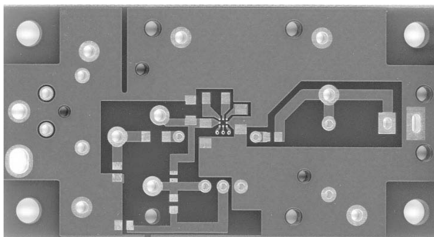
Layer 2 wiring
