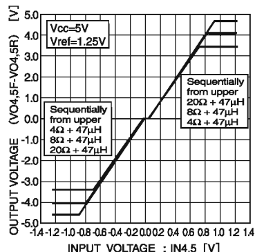
Fig. 21 CH 4 , 5 l / O characteristic : Ta=90°C
