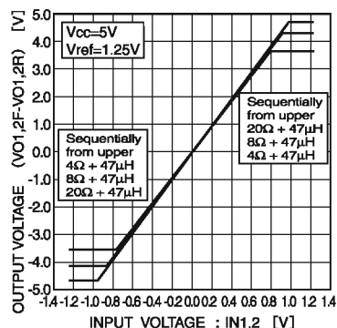
Fig. 15 CH 1,2 / O characteristic : Ta=90°C
