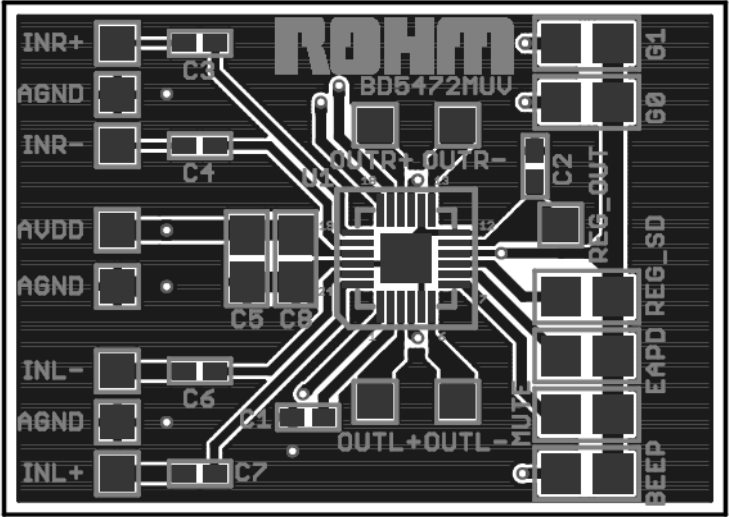
Top Layer
