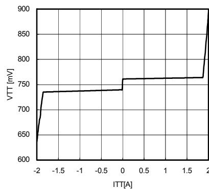
Fig.6 ITT-VTT (DDR3)
