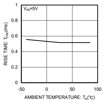
Fig.19 Output rise time
