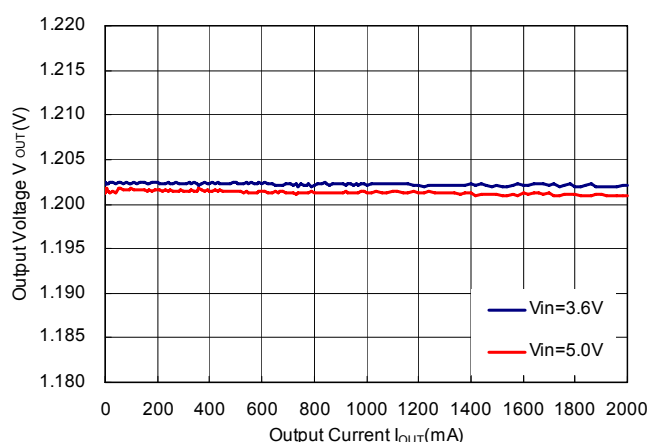
RP506Kxx1D/E/F V_{OUT}=1.2V
