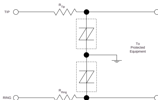
FIGURE 2 - Longitudinal Protection
