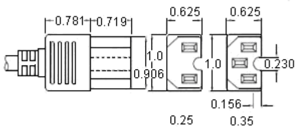
Dimensions : Millimetres
