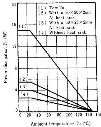
P_D - T_a (PU3219)
