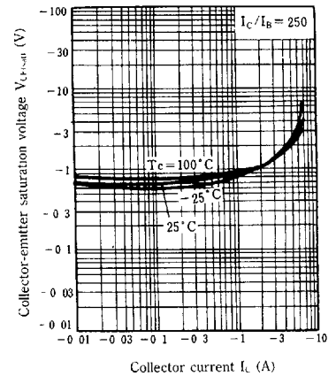
V_{CE(sat)} - I_C
