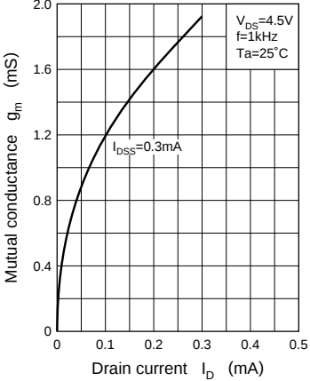
g_m - I_D
