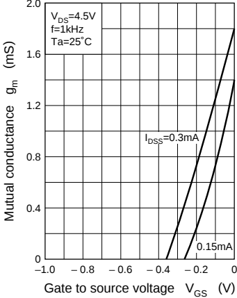
g_m - V_{GS}
