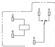
端子排列/外部接口 (BOTTOM VIEW)
