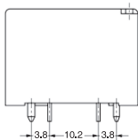
端子排列/外部接口 (BOTTOM VIEW)
