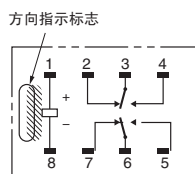
端子配置/内部连接图 (BOTTOM VIEW)
