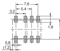
印刷基板加工尺寸 (TOP VIEW) 尺寸公差±0.1mm
