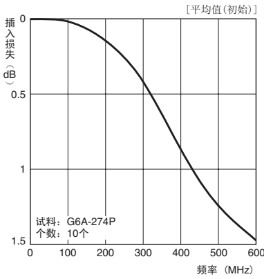
高频特性（插入损失） *1、*2
