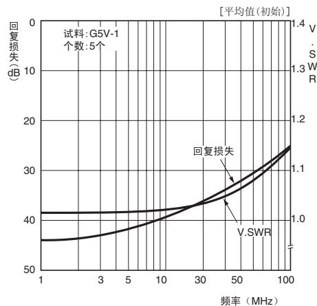
高频特性（回复损失、V.SWR）*1、*2
