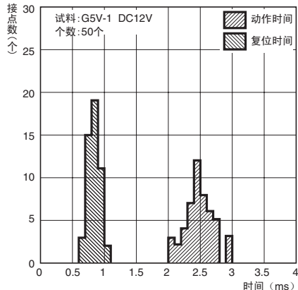
动作・复位时间的分布*1
