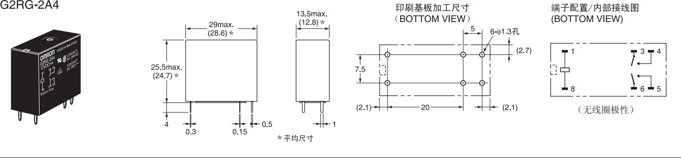
G2RG-2A4
