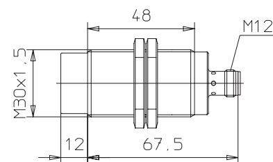
E2EL-X15M□-M1L
