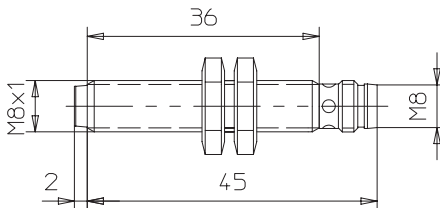
E2EL-X2M□-M3
