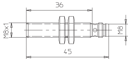
E2EL-X1R5□-M3
