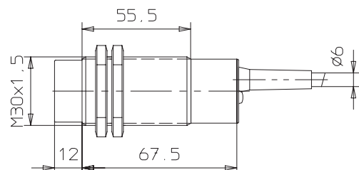
E2EL-X10□-L 2M
