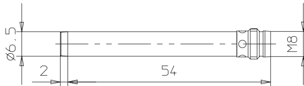
E2EL-C2M□-M3L
