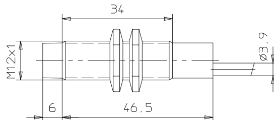
E2EL-X4M□-L 2M
